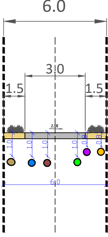
ПОПРЕЧНИ ПРОФИЛ
