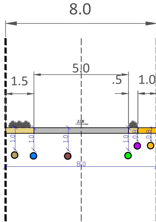
ПОПРЕЧНИ ПРОФИЛ
