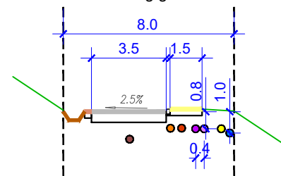
ПРИСТУПНИ ПУТ У НАЦИОНАЛНОМ ПАРКУ ДО МАНАСТИРА 3-3
