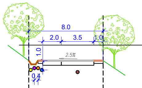
ПРИСТУПНИ ПУТ У НАЦИОНАЛНОМ ПАРКУ 5-5
