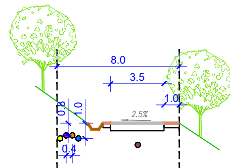
ПРИСТУПНИ ПУТ У НАЦИОНАЛНОМ ПАРКУ 6-6
