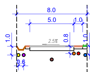
ПРИСТУПНИ ПУТ У ЗОНИ КУЋА ЗА ОДМОР 4-4
