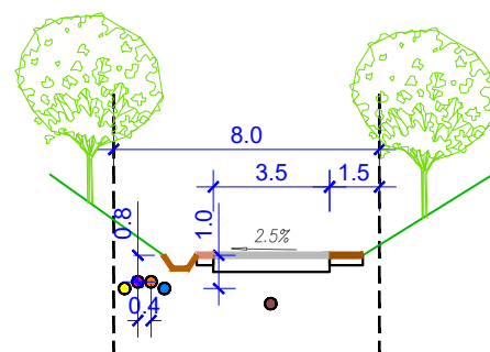
ПРИСТУПНИ ПУТ У НАЦИОНАЛНОМ ПАРКУ 7-7
