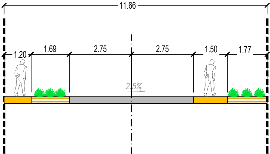
ПОПРЕЧНИ ПРОФИЛ 2-2
