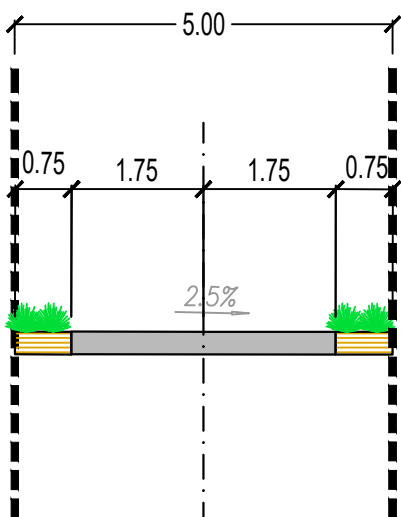
ПОПРЕЧНИ ПРОФИЛ 4-4
