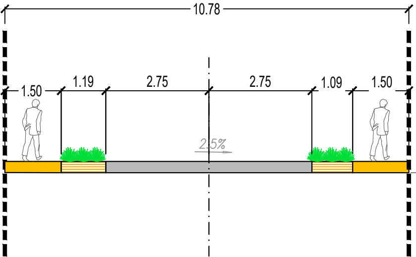
ПОПРЕЧНИ ПРОФИЛ 1-1
