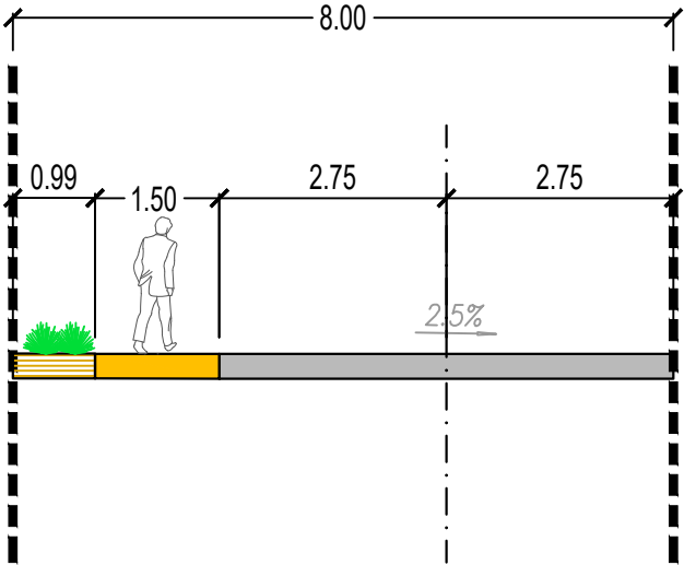
ПОПРЕЧНИ ПРОФИЛ 3-3
