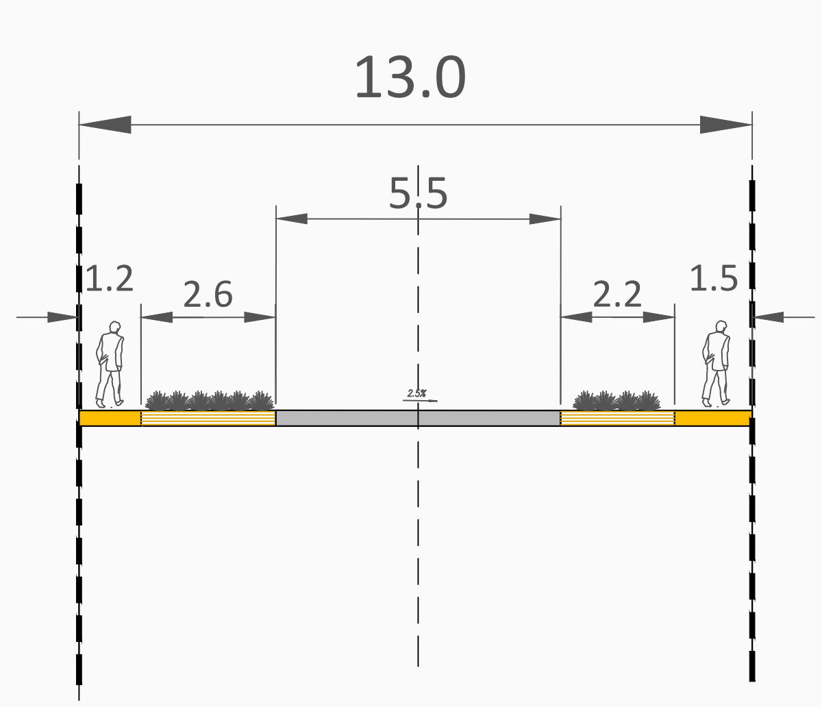
ПОПРЕЧНИ ПРОФИЛ 1-1
