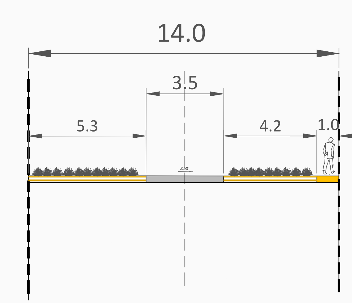
ПОПРЕЧНИ ПРОФИЛ 3-3
