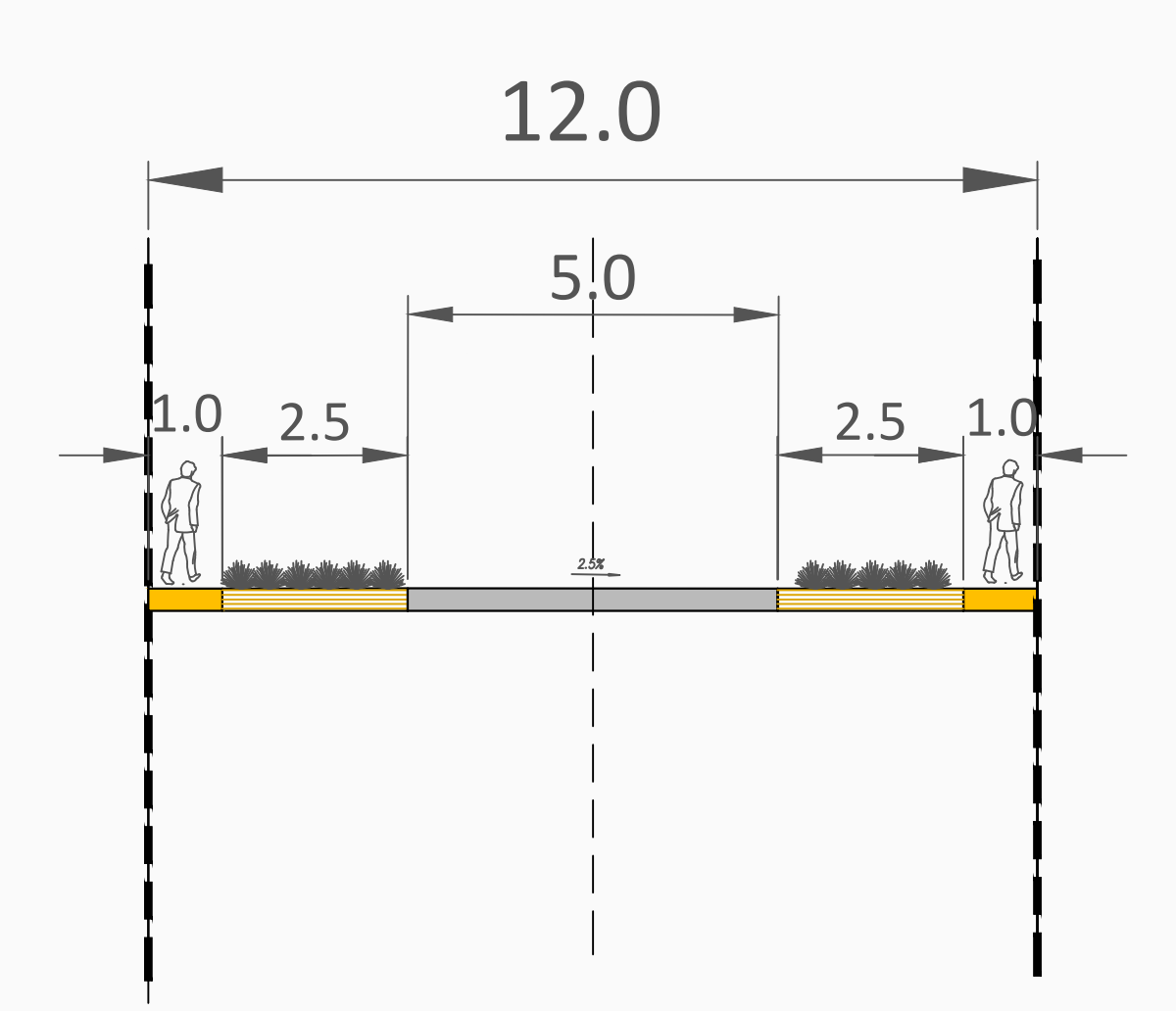
ПОПРЕЧНИ ПРОФИЛ 2-2
